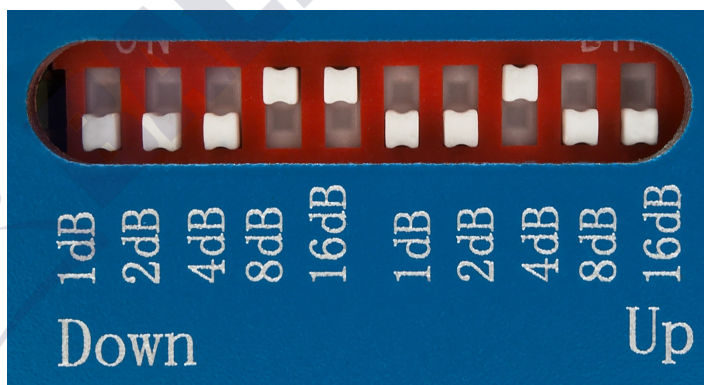
Ручная регулировка усиления. Положение «вверх» — включено, положение «вниз» — выключено
