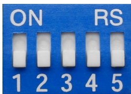
Ручная регулировка усиления. Положение переключателей «вверх» — включено, положение «вниз» — выключено
