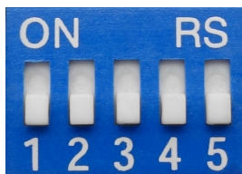
Ручная регулировка усиления. Положение переключателей «вверх» — включено, положение «вниз» — выключено
