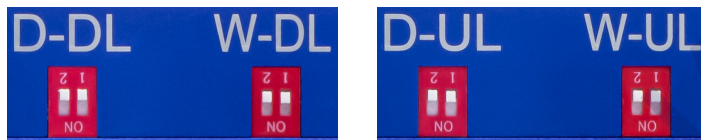
Ручная регулировка усиления. Положение переключателей «вверх» — выключено, положение «вниз» — включено
